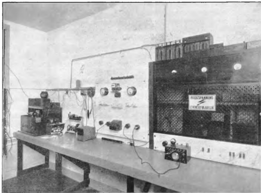
EEN HOEKJE VAN ONS LABORATORIUM. — Rechts hoogspanningkast met krachtversterker, de microfoonversterker staat op den voorgrond. De op het schakelbord zichtbare meters registreren het stroomverbruik der aangesloten apparaten, die op verschillende groepen ingeschakeld worden. De gelijkstroomaansluiting met een bedrijfsspanning van ruim 700 volt is op deze foto juist zichtbaar.
